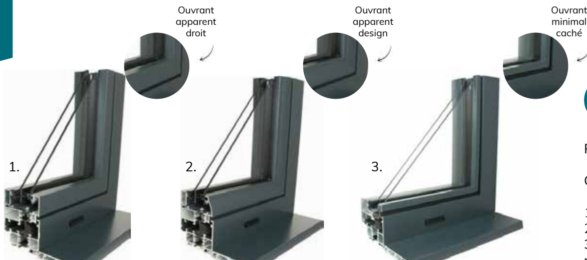
Rupture de pont thermique pour une isolation maximale - Double vitrage 6/14/4 à isolation renforcée
