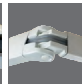
Bras à chaînes à rouleaux. Testés à 20 000 cycles.
