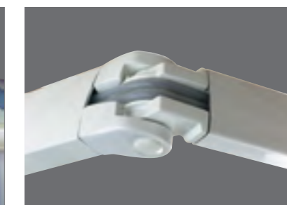
Bras à double câbles gainés testés à 20 000 cycles.
